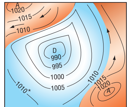
(D) : Depression (A) : Anticyclone
